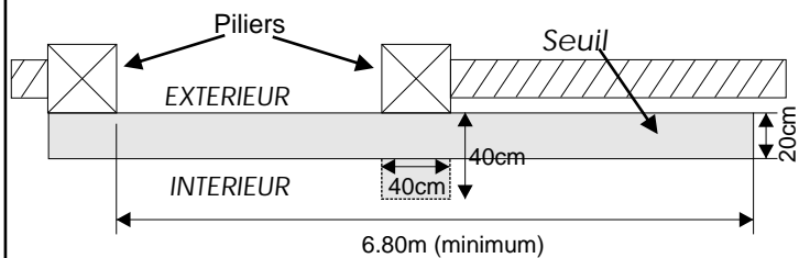
(Vu de dessus) ouverture vers la gauche (vu depuis l'extérieur)
