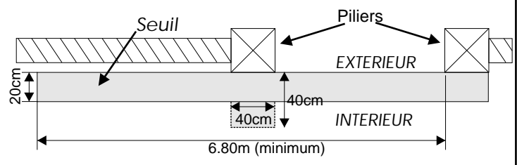
(Vu de dessus) ouverture vers la droite (vu depuis l'extérieur)
